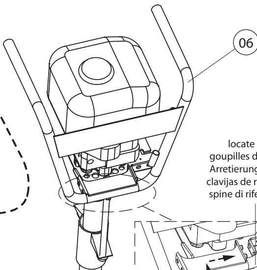
FIG. 4 MOVING THE MAIN HANDLE DÉPLACEMENT DE LA MANETTE DREHUNG DES HALTEGRIFFES DESPLAZAMIENTO DE EL BRAZO SPOSTAMENTO DEL MANUBRIO
